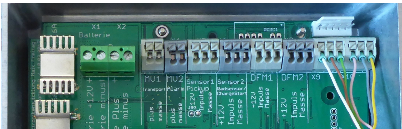
Abbildung 2: Kommunikationsanschluß SEQU-BT
