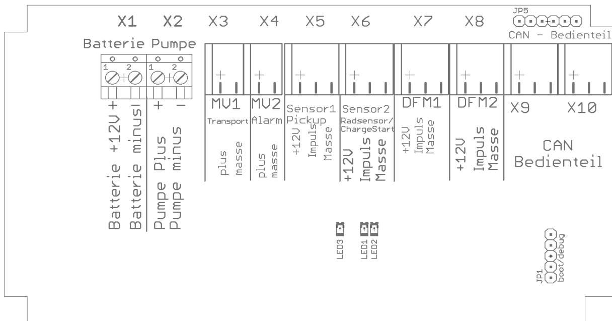
Abbildung 1: Klemmenbelegung SEQU-LT-12/150
