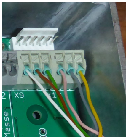
Abbildung 2: Kommunikationsanschluß zum Bedienteil SEQU-BT
