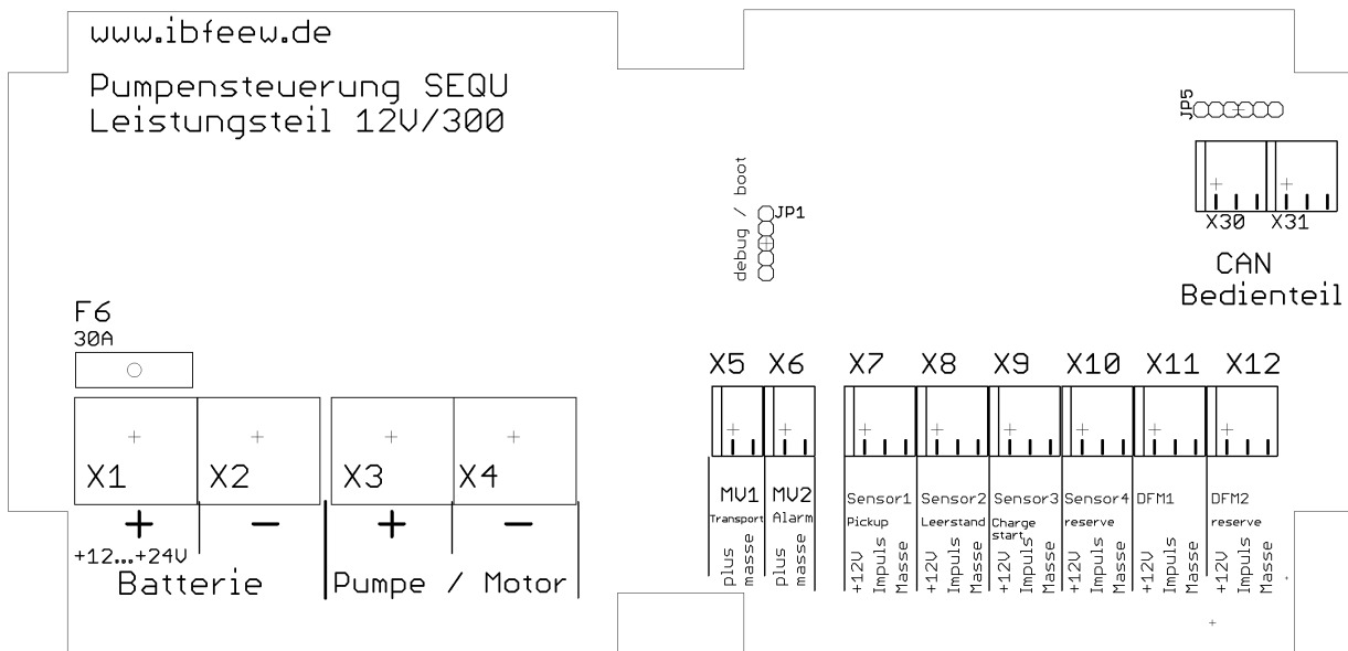
Abbildung 1: SEQU-LT12V/300: Anschlußklemmen
