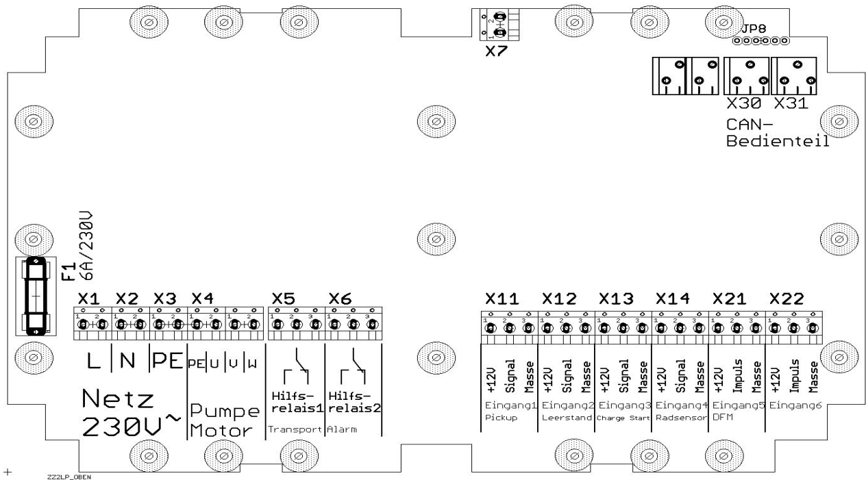
Abbildung 1: SEQU-LT12/050: Anschlußklemmen
