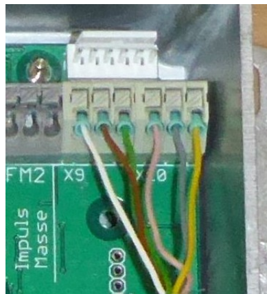
Abbildung 3: Anschluß Verbindungskabel zum Bedienterminal
