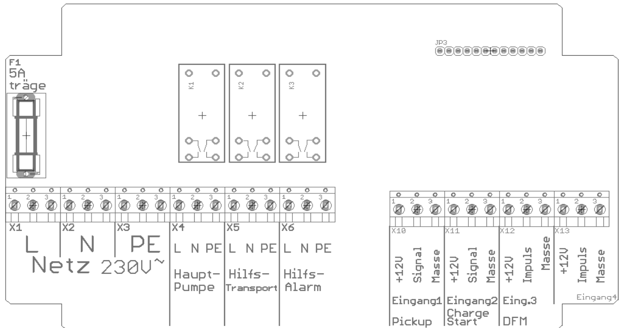
Abbildung 1: Anschlußklemmen SEQU-Switch-mini
